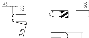
라운드레일 SCALE: NONE
