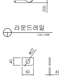
사각와셔 SCALE: NONE
