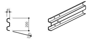
레일 상세도
