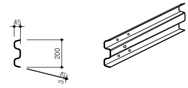
레일 상세도
