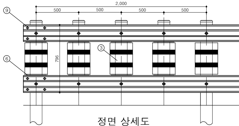
정 면 도(S=1/2)
