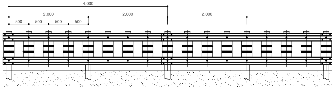
정 면 도(S=1/2)
