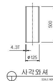
사각와셔 SCALE: NONE
