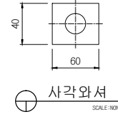
사각와셔 SCALE: NONE
