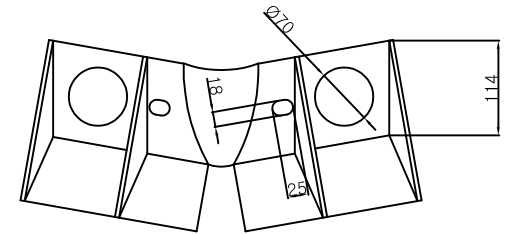
브라켓상세도
