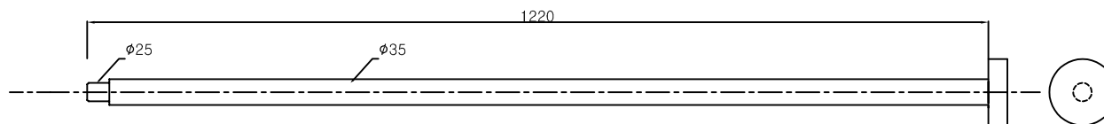
항타봉
