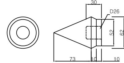
뺨기 상세
